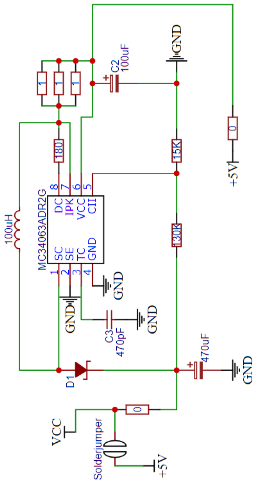
Obrázek A.3: Úplné schéma obvodu step-up převodníku z 5 na 12 voltů. Obvod zahrnuje nula ohmové odpory a solder jumper, které umožňují jednoduché odpojení převodníku.
