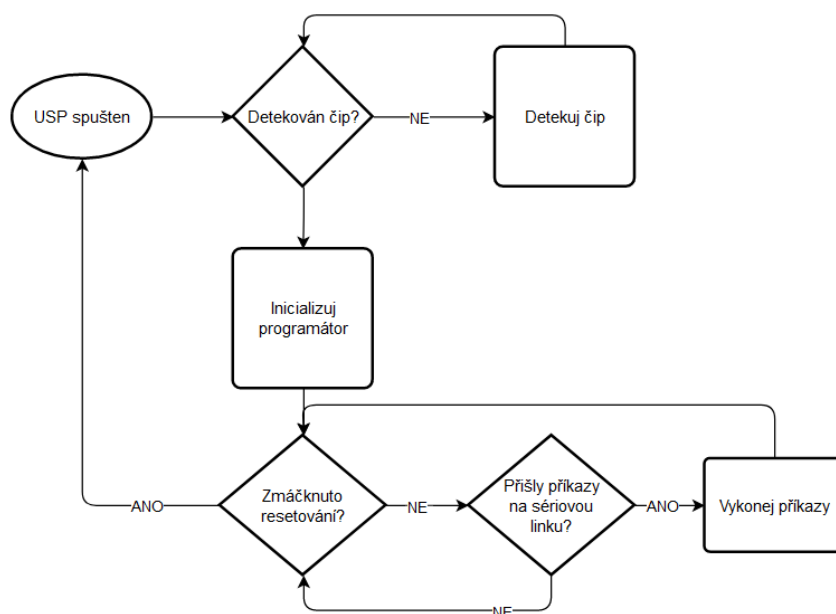
Obrázek 2.4: Diagram USP
