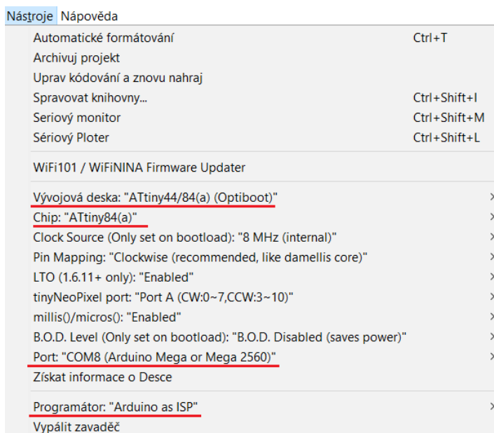
Obrázek 3.2: Nastavení Arduino IDE pro nahrávání do čipu ATtiny84; zvýrazněny jsou nejdůležitější parametry.
