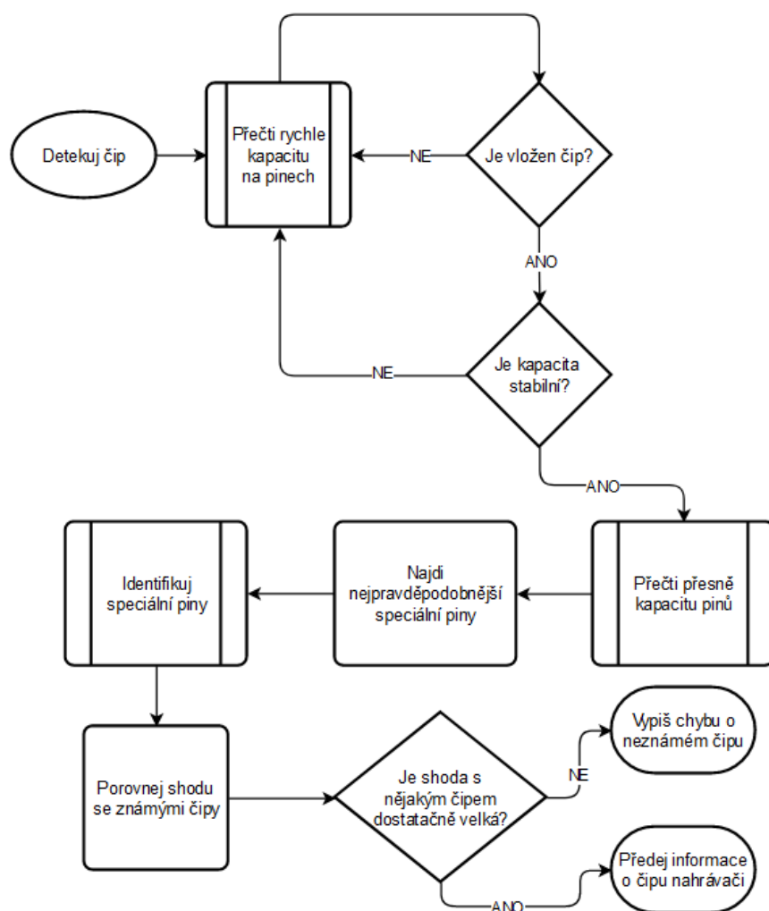
Obrázek 2.5: Diagram fungování detektoru. Dvojité obdélníky značí funkce, které interagují s hardwarem
