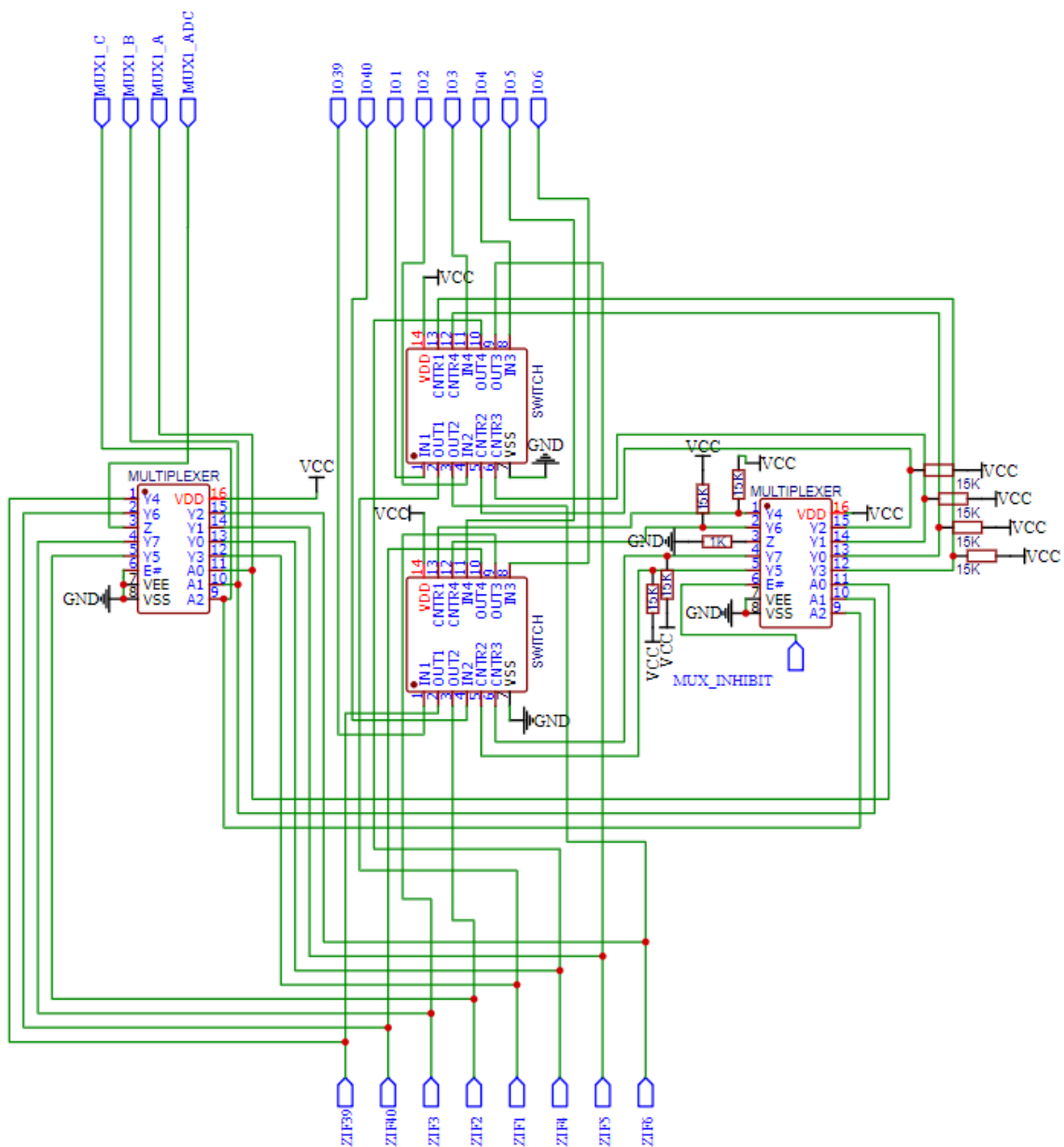
Obrázek A.1: Úplné schéma obvodu připojeného k 8 pinům ZIF patice.
